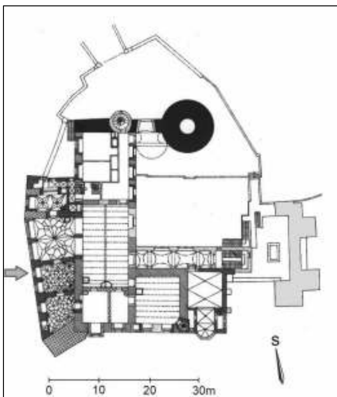
Obr. 19. Hrad Šternberk – půdorys prvního patra s vymezením jednotlivých stavebních fází. Berkovský trakt značen šipkou (Převzato z Vítek, Tomáš: Válcová věž šternberského hradu . In: Sborník Národního památkového ústavu územního odborného pracoviště v Olomouci. Olomouc 2010, s. 136).
